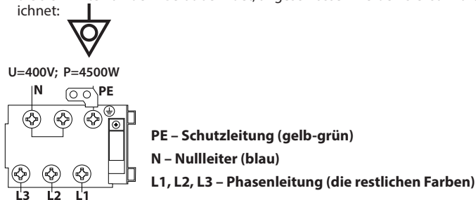
Abb. 2 - Etikette mit dem Schaltplan
